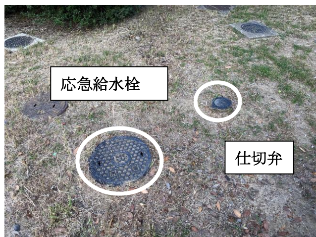
応急給水栓の設置状況
