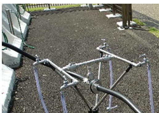
② 連結部品とホースを接続
