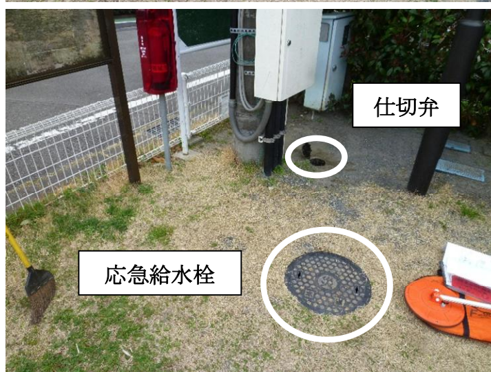
【詳細図】
